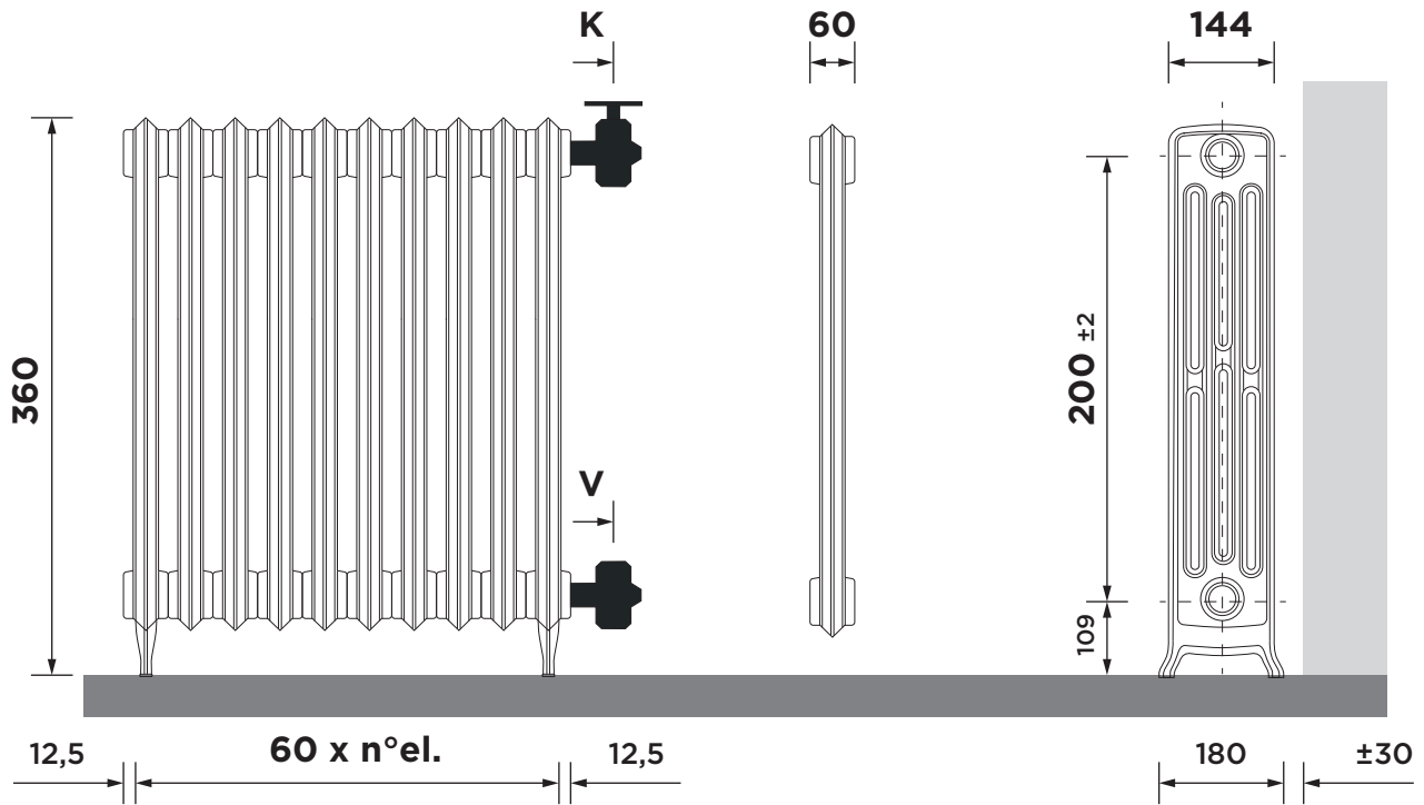
on the floor | bodenstehend | vloerstaand | на зemi | на полу/ногах BI4/360-F, all dimensions in mm ±2
