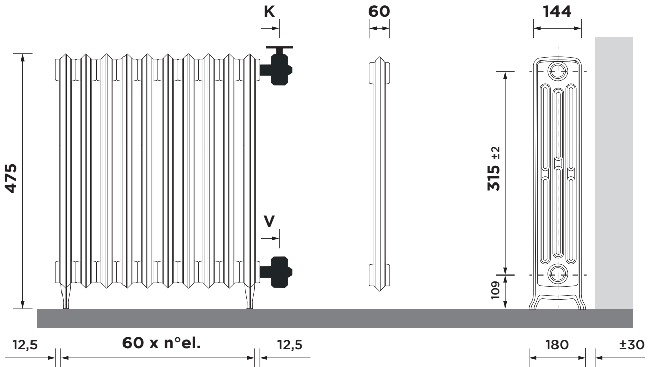
on the floor | bodenstehend | vloerstaand | на зemi | на полу/ногах BI4/475-F, all dimensions in mm ±2
