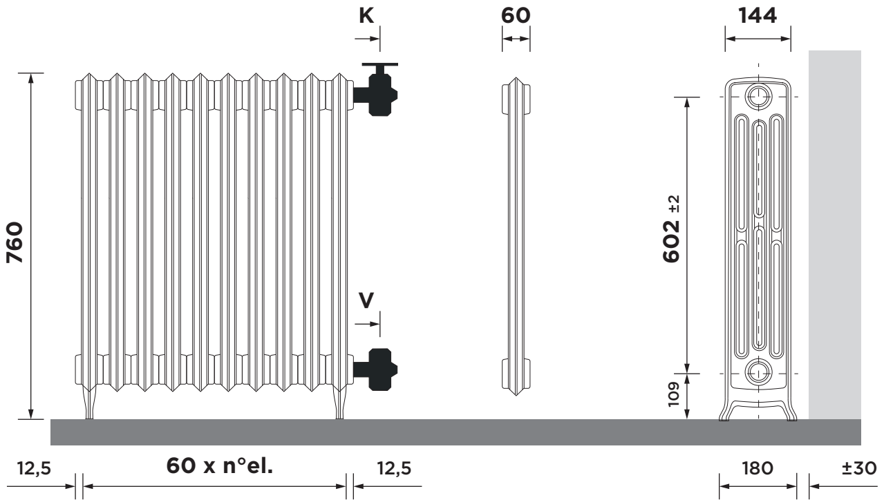
on the floor | bodenstehend | vloerstaand | на зemi | на полу/ногах BI4/760-F, all dimensions in mm ±2
