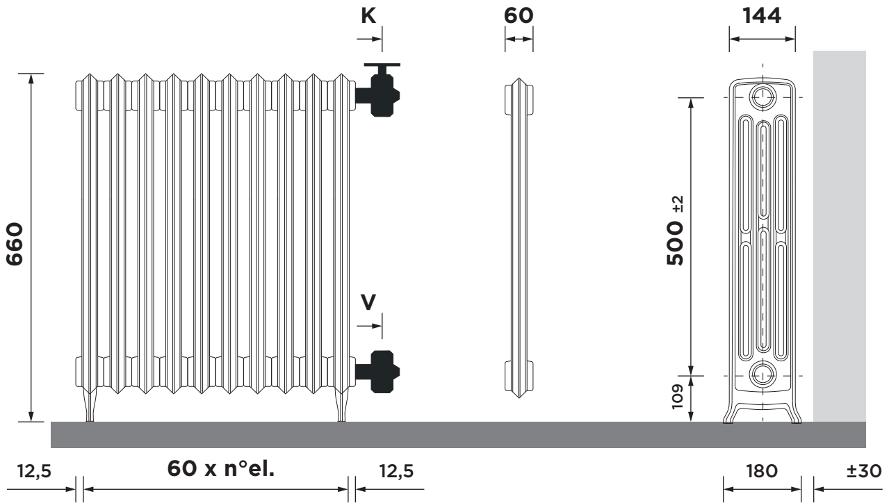
on the floor | bodenstehend | vloerstaand | на зemi | на полу/ногах BI4/660-F, all dimensions in mm ±2
