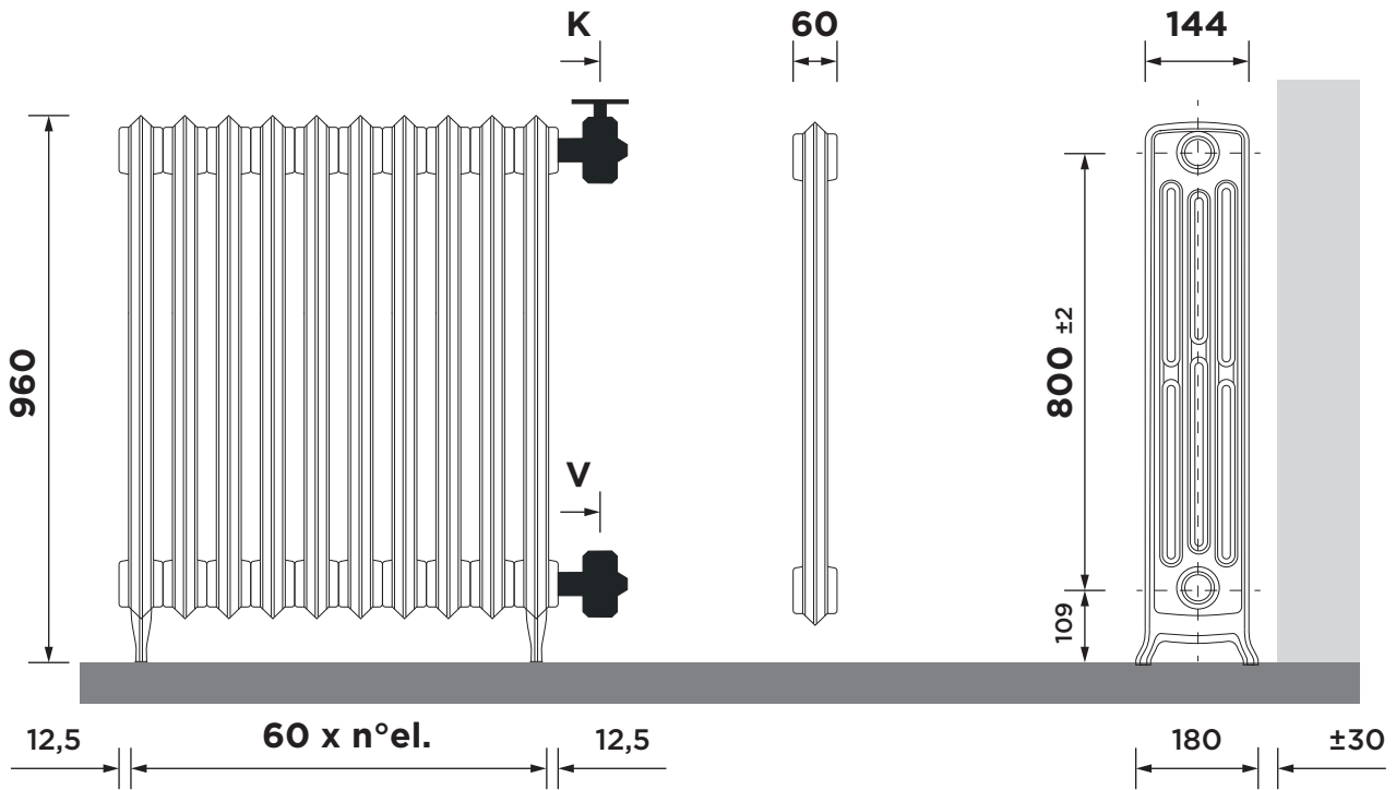
on the floor | bodenstehend | vloerstaand | на зemi | на полу/ногах BI4/960-F, all dimensions in mm ±2
